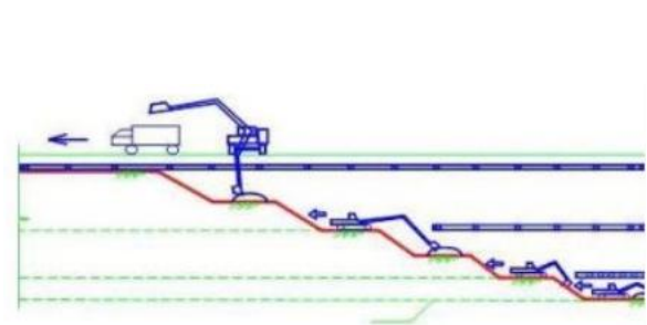
严格按设计和施工方案的要求分层、分段开挖且均衡开挖
