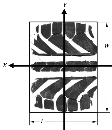
图 1 接触区域印痕
