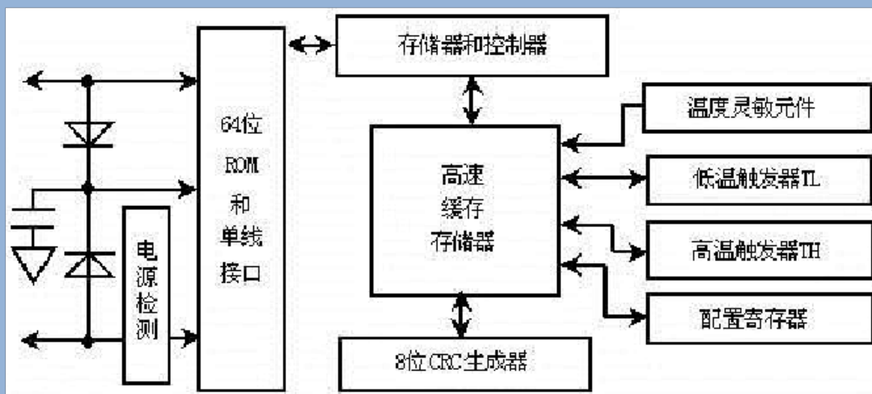
图3 DS1820的内部框图
