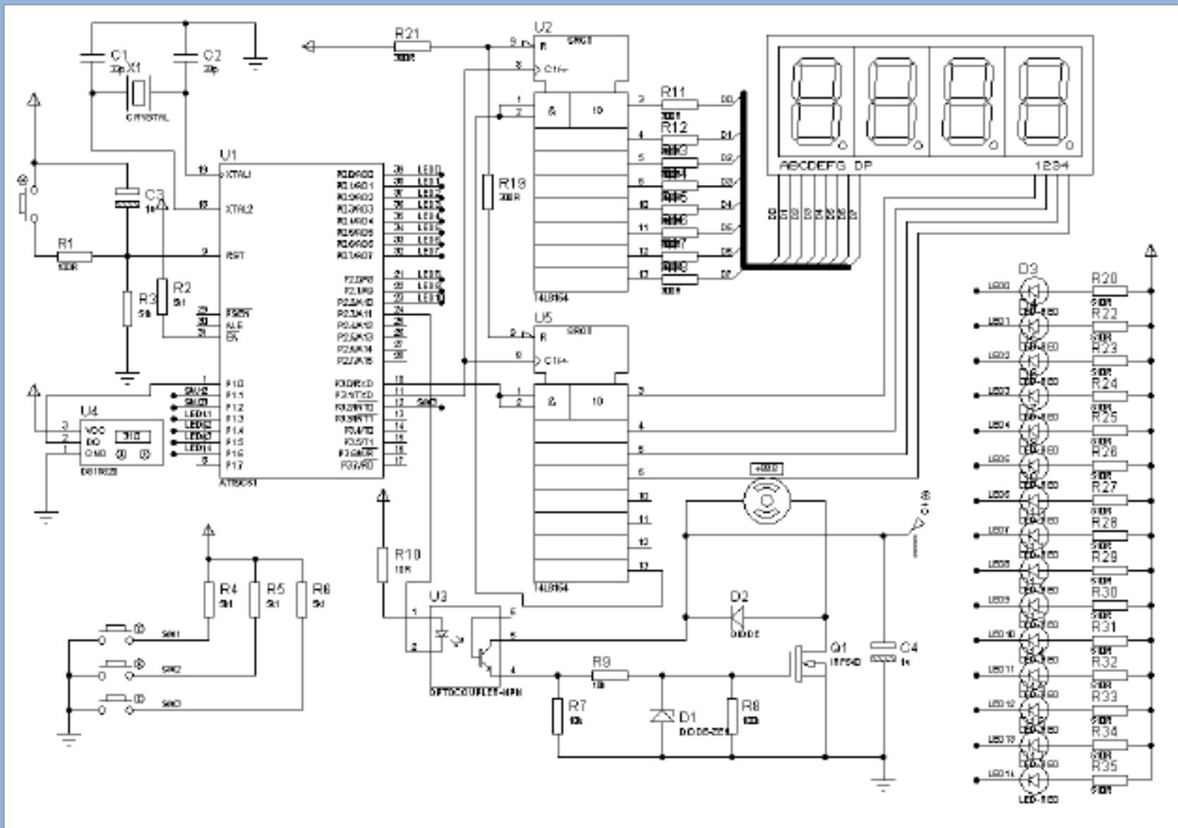
图 2 智能温度测量系统原理图
