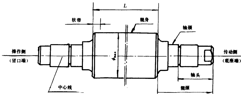
轧辊示意图
