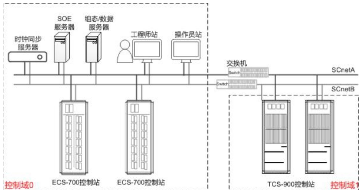
图 1-1 TCS-900 系统集成到 ECS-700 系统的典型组网图
