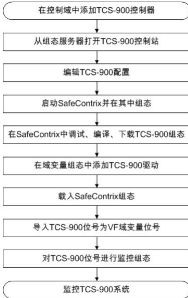
图 3-1 TCS-900 系统集成到 VF 软件的操作流程图
