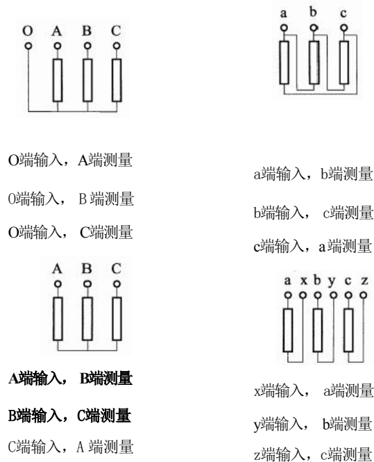
图2 变压器常用检测接线方式
