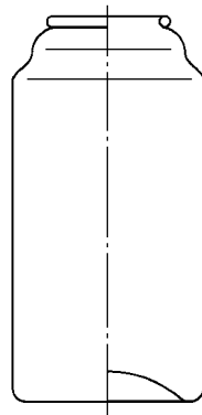
图 1 铝气雾罐
