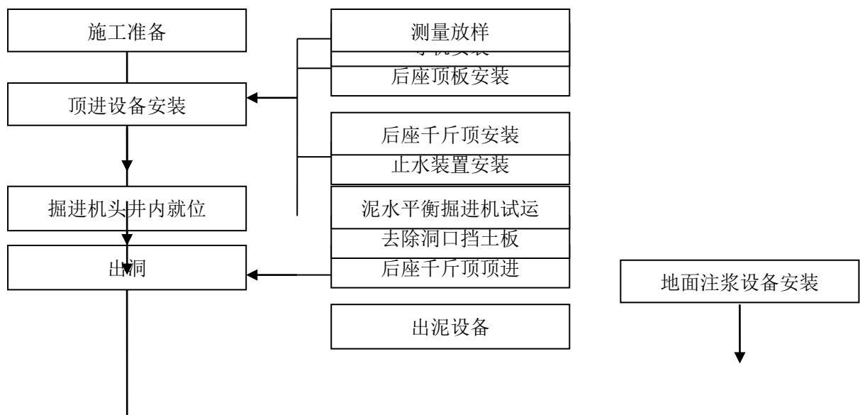
顶管施工工艺流程图
