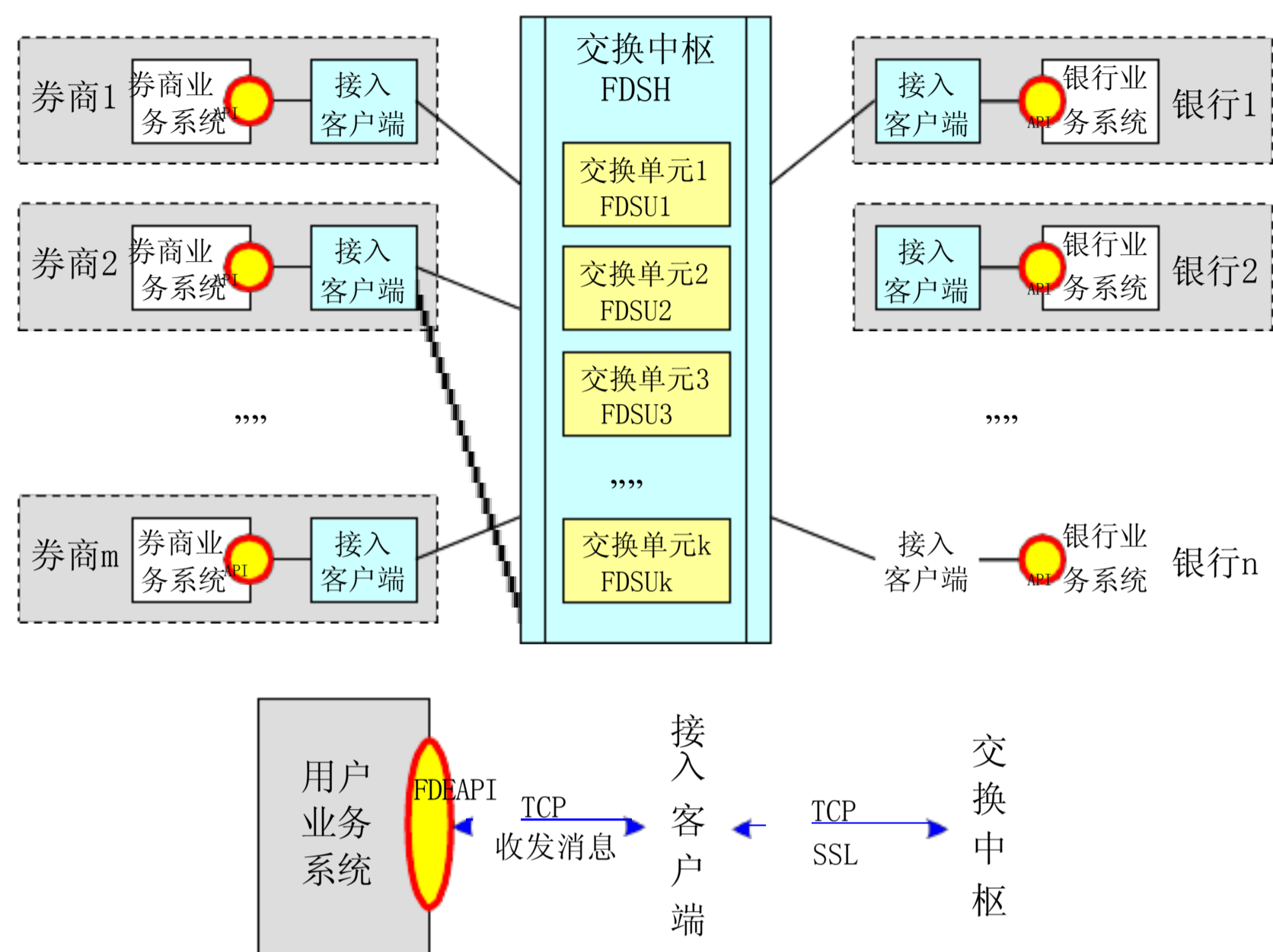
图1 FDEAPI应用环境
