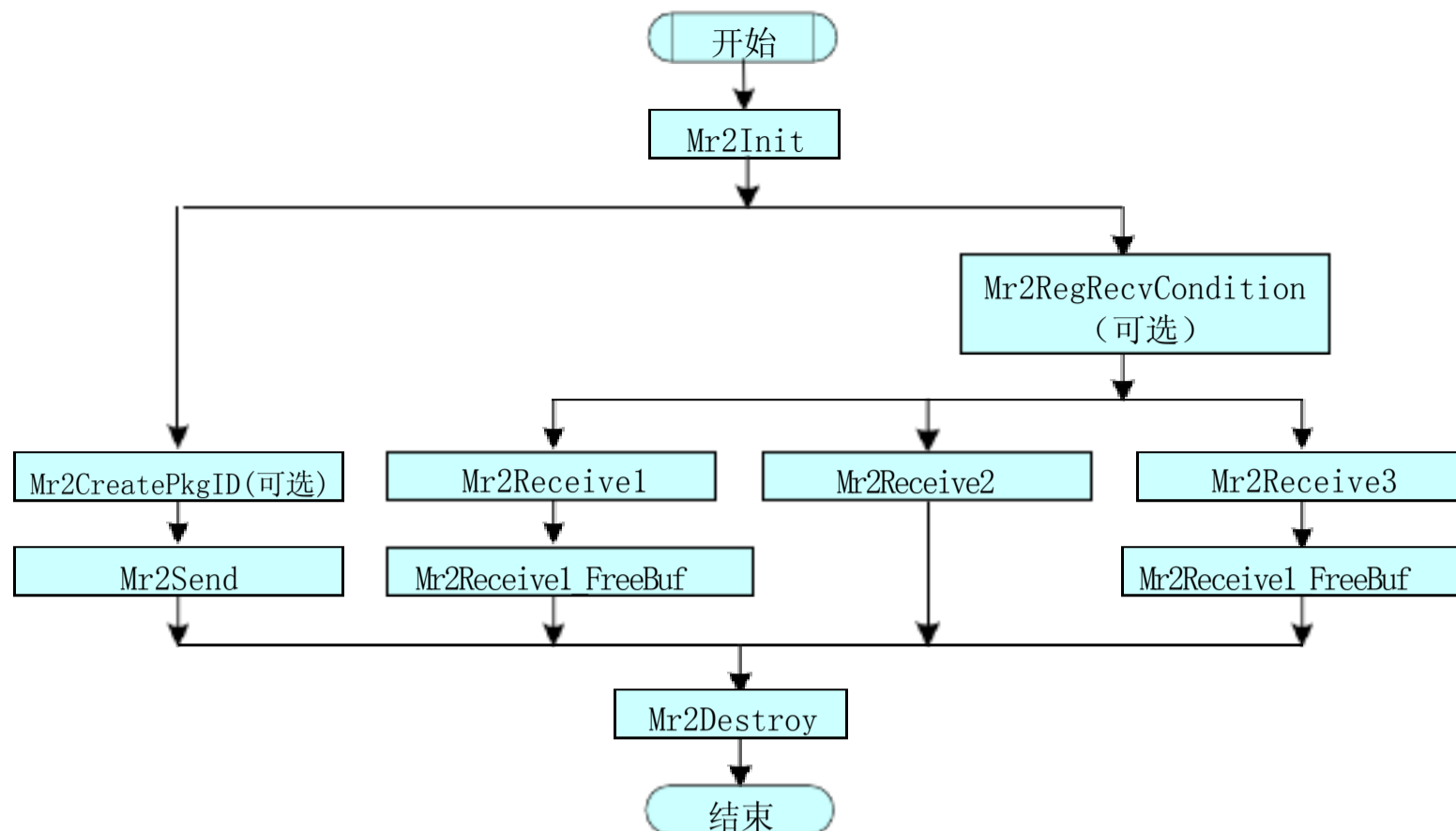
图3 FDEAPI主要函数调用顺序
