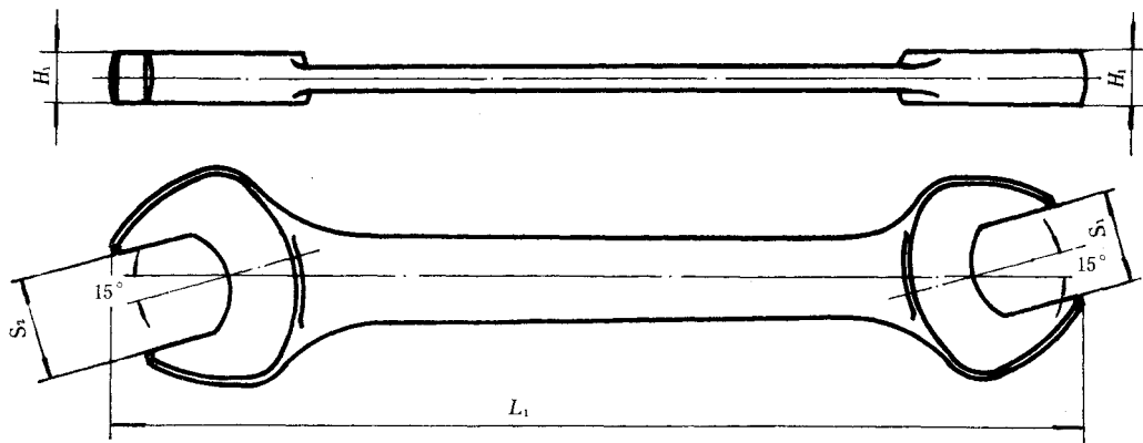
图 1 双头呆扳手
