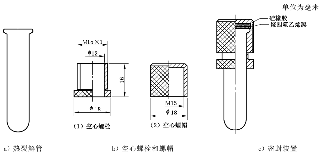
图 1 热裂解管及密封装置
