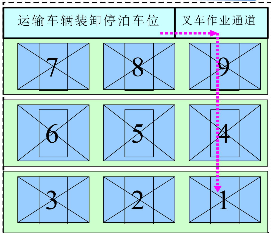
拣货区布局图
