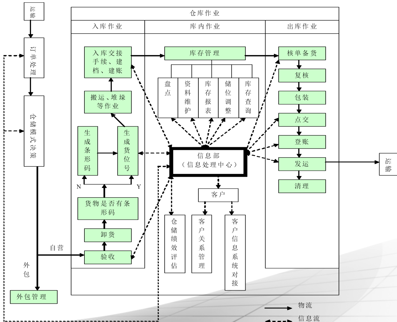
图 2-8 重组后的仓储流程
