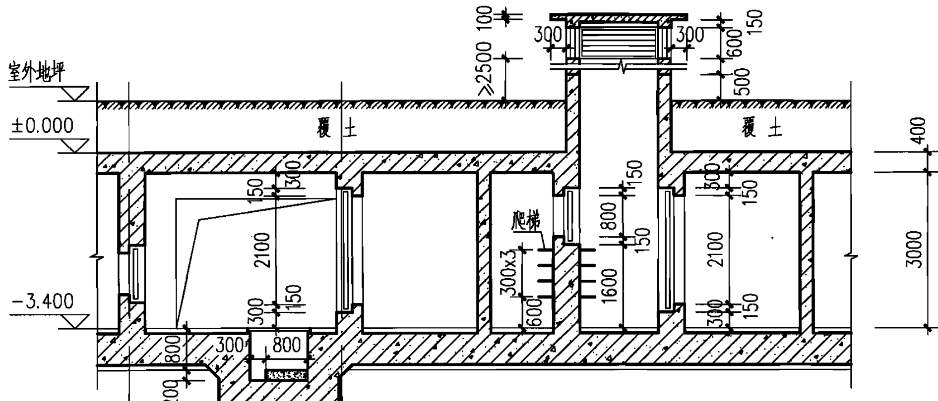
1-1 剖面图
