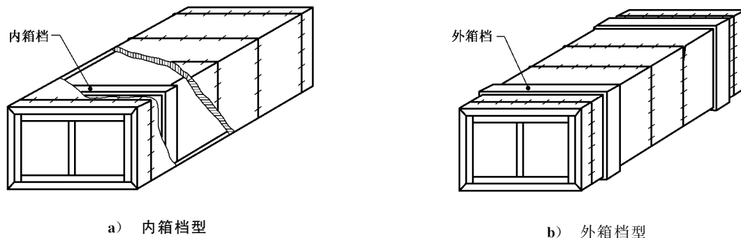
图 1 箱档的结构示例
