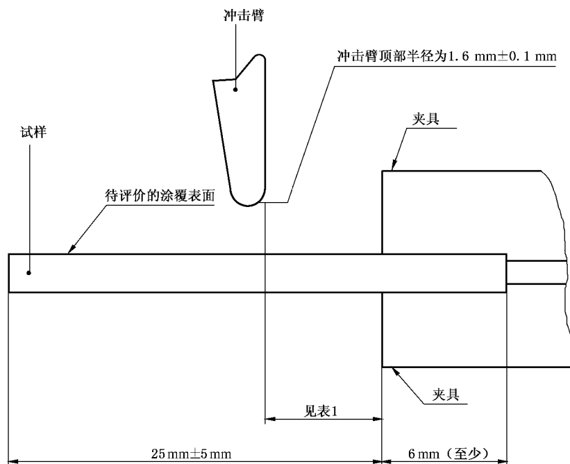
图 1 试样夹具和冲击臂
