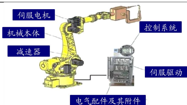
图2 工业机器人关键零部件
