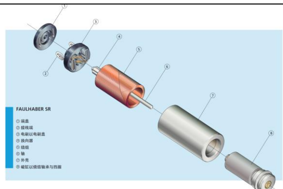
图16 有刷空心杯电机
