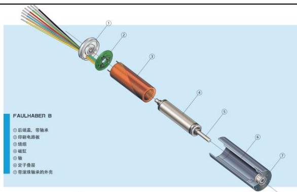
图15 无刷空心杯电机
