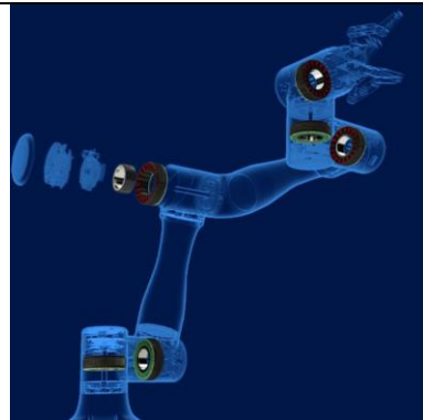
图14 协作机器人和关节模组 (采用无刷力矩电机)
