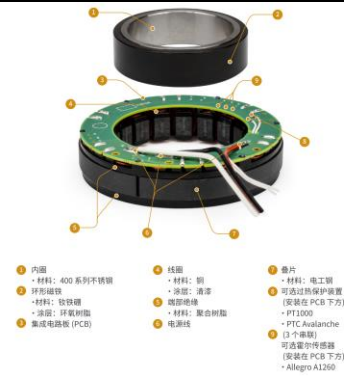
图12 科尔摩根无刷电机组成
