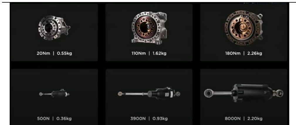
图10 特斯拉“擎天柱”执行器
