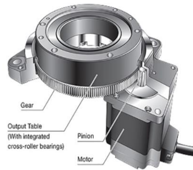
图9 旋转执行器示意图
