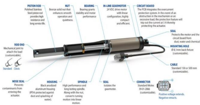
图8 线性执行器示意图
