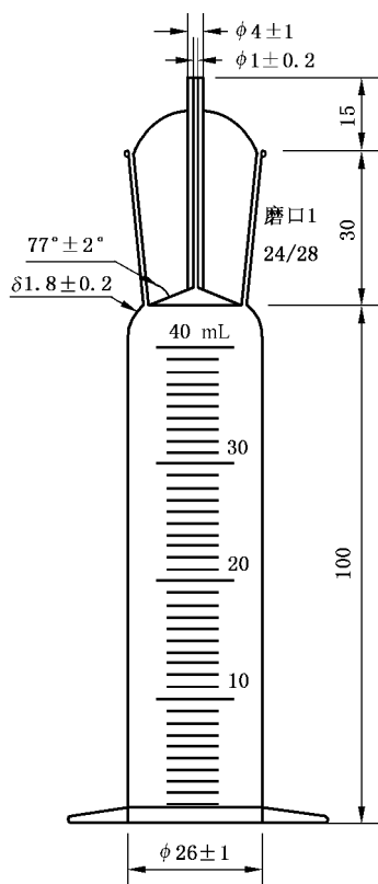
图 1 离子交换树脂密度计
