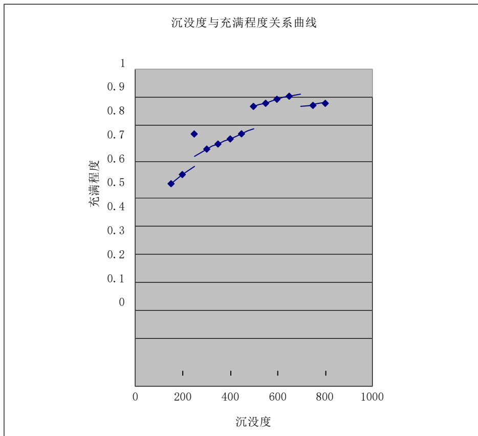
充满程度与沉没度的关系曲线
