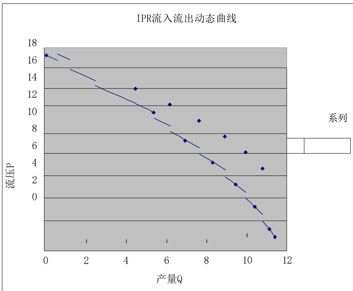
— IPR曲线 (图1) —
