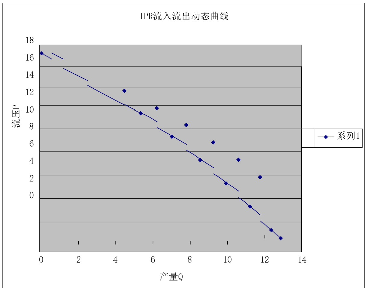
IPR曲线
