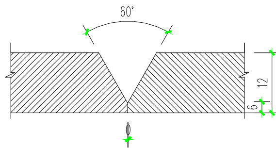
直缝焊坡口形式
