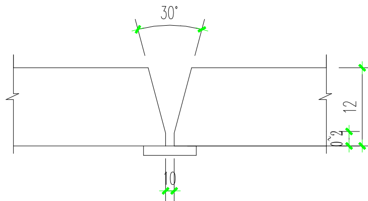
钢管对接焊坡口形式
