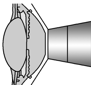
图 1 压平眼压计测量示意图
