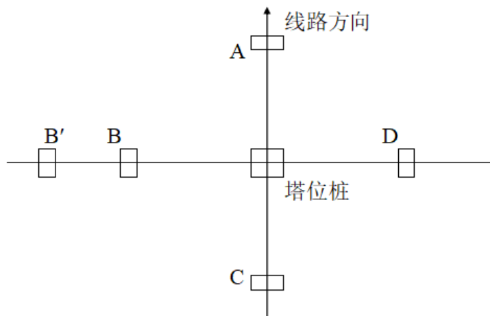
图 5.1.3-2 定直线杆塔的辅助桩图
