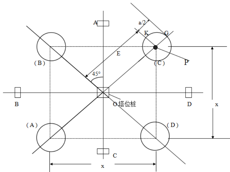
图 5.1.3-3 中心桩至基础坑中心距离
