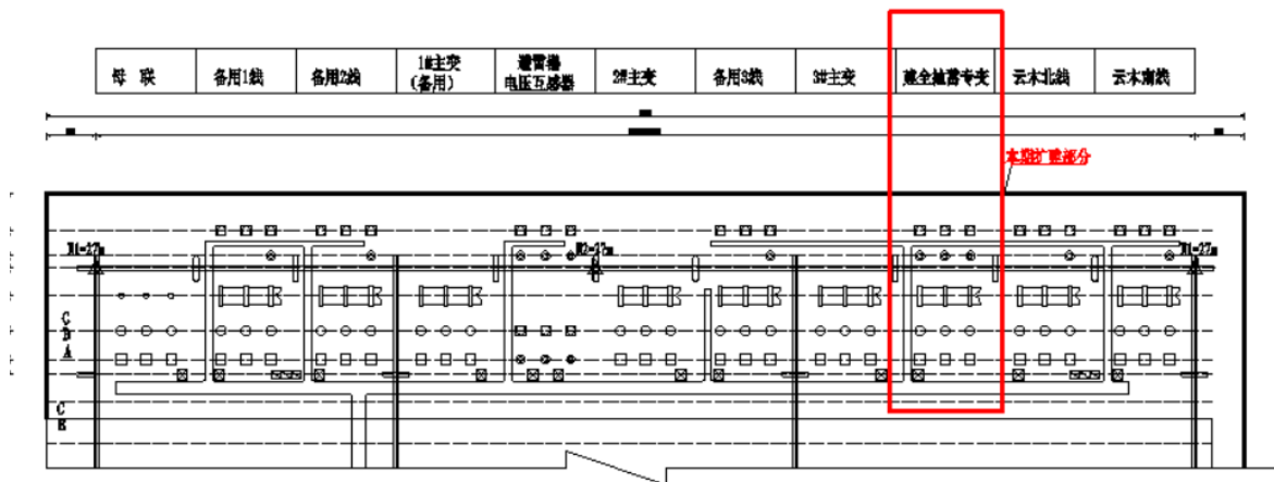
图 1.1.1-1 110kV 变电站平面布置图
