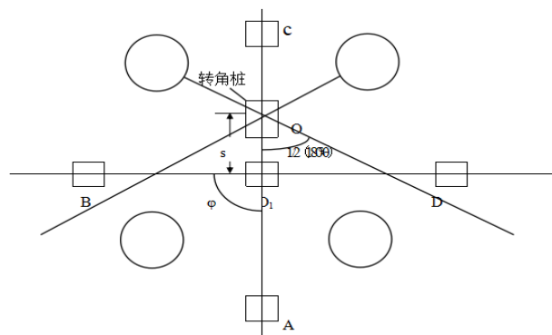
图 5.1.3-4 位移转角塔分坑图
