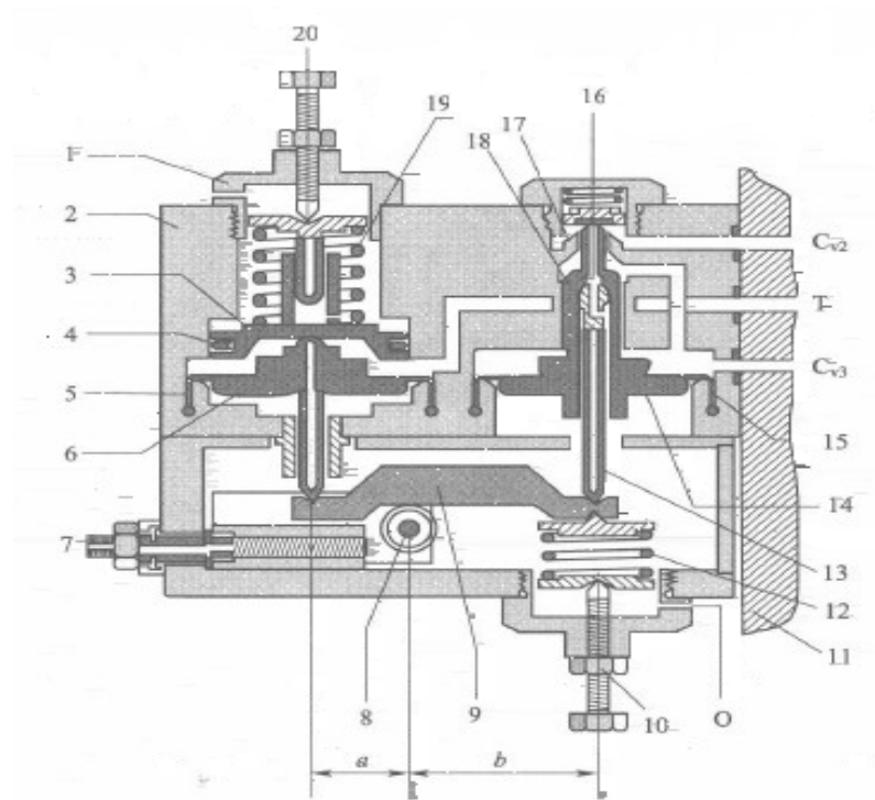
图 2.4 称重阀
