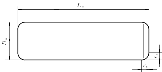
图 1 平头滚针
