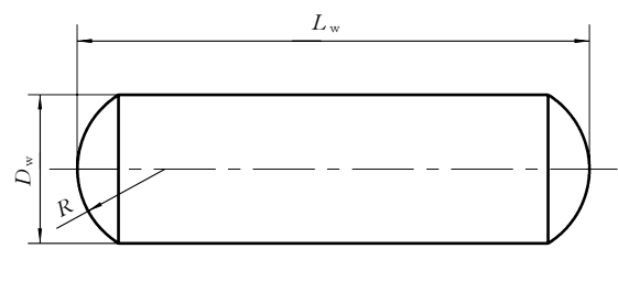
图 2 圆头滚针
