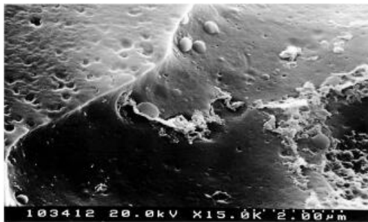
光敏技术网点与边缘热敏技术网点边缘
