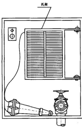
图 4 托架式栓箱
