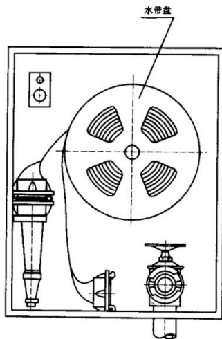
图 2 盘卷式栓箱
