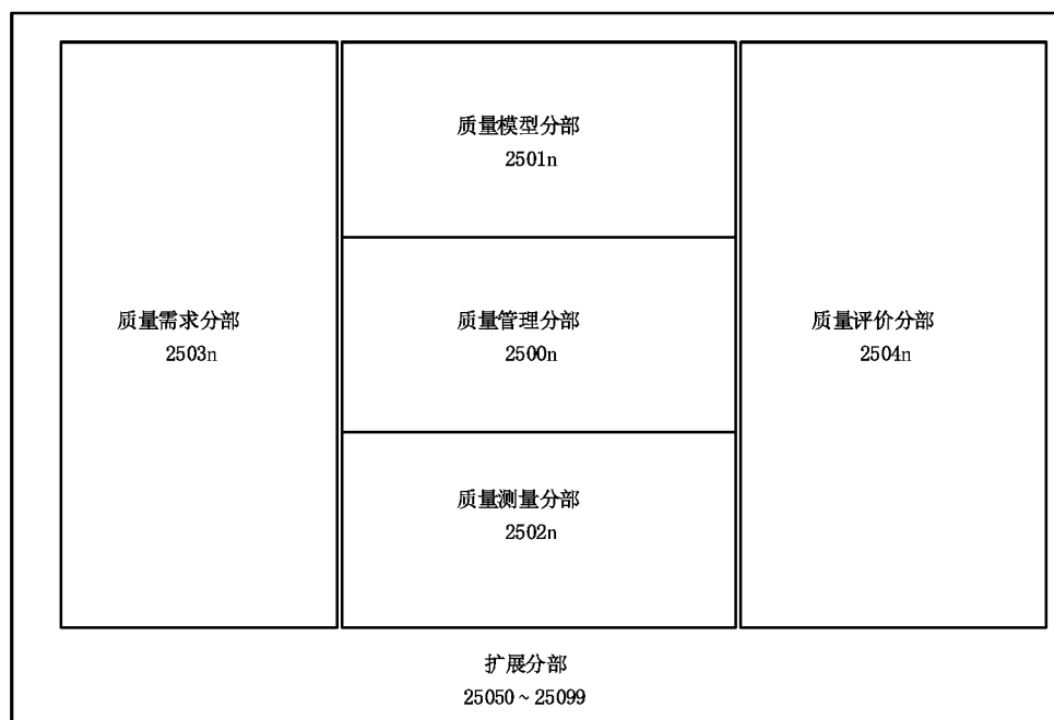
图 1 SQaRE 系列标准组织结构
