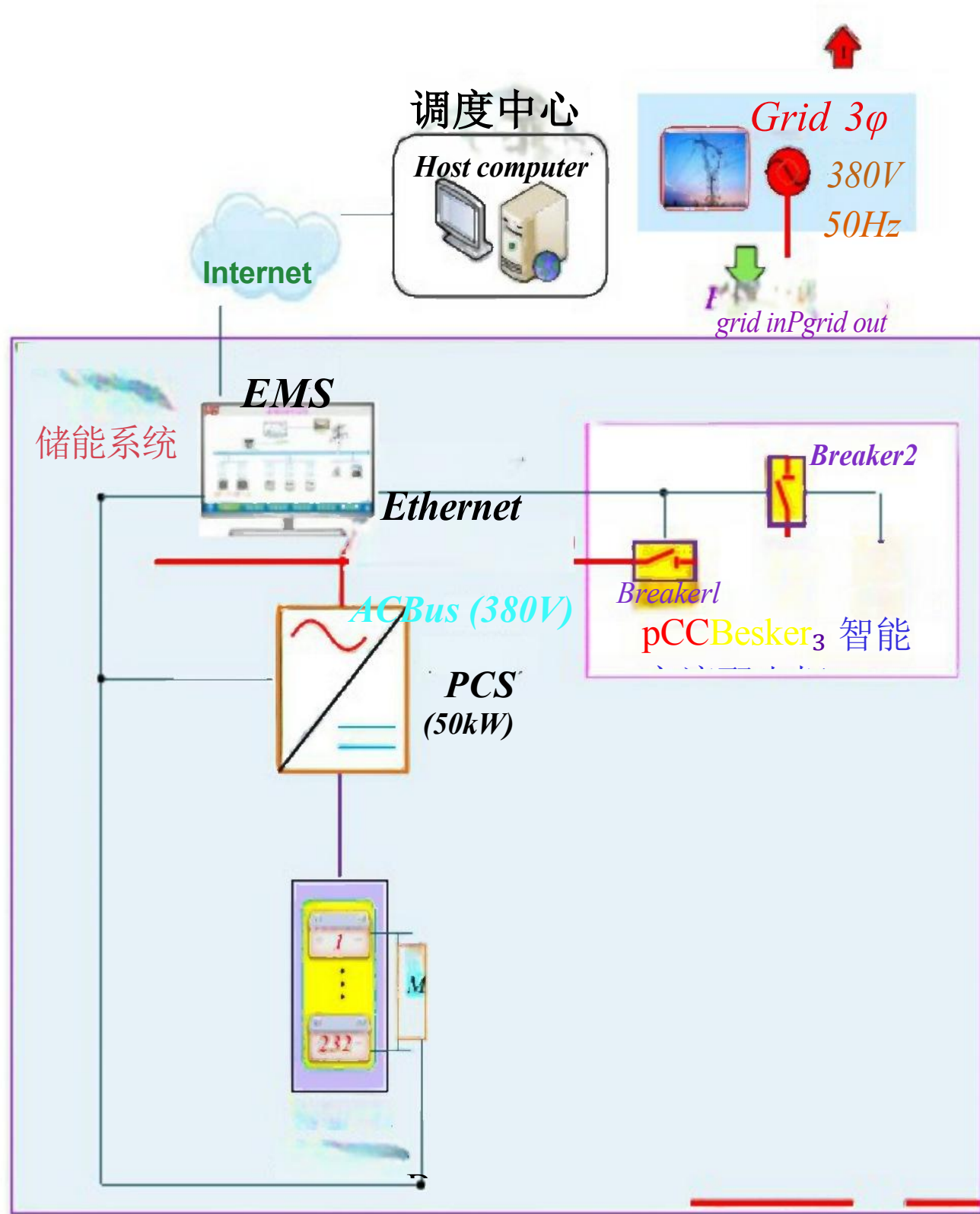
图 3 5 0kWh集装箱式储能系统拓扑
